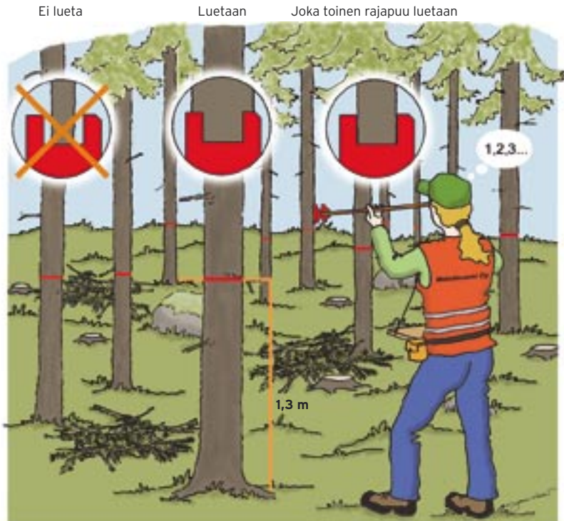
Kuva 8. Puiden lukuperiaate relaskooppilla. Hahlon täyttävät puut luetaan pohjapinta-alaan. Jos rajaetäisyyttä ei tarkasteta, joka toinen rajapuu luetaan mukaan.
