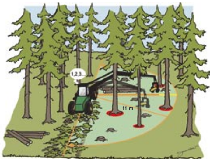
Kuva 5. Koneenkuljettaja voi seurata harvennusvoimakkuutta ajouralta käsin lukemalla puoliympyrän sisään jäävät puut ja vertaamalla tulosta keskiläpimittaan perustuvaan harvennusmalliin.
